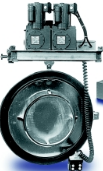
Recirc Nozzle Plug
